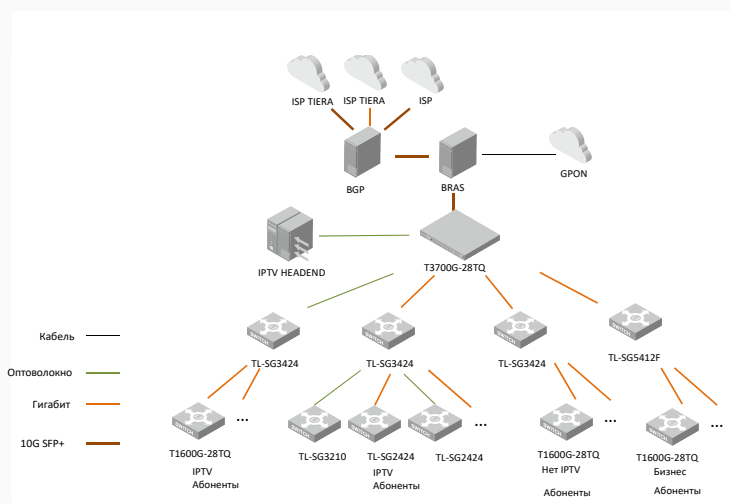
Топология сети Citynet
